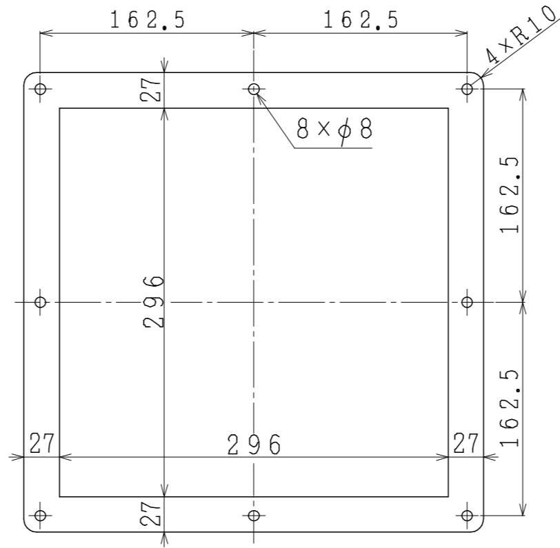
A-B矢视图
