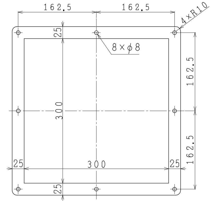
C-D矢视图
