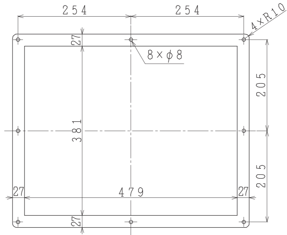
E-F 矢視図
