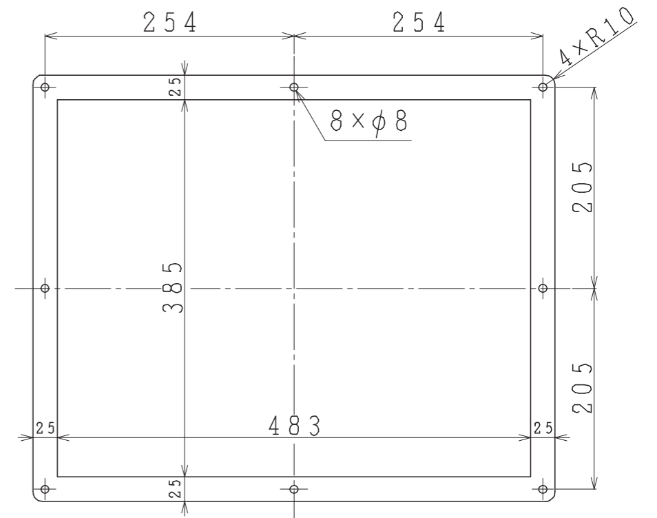
G-J 矢視図
